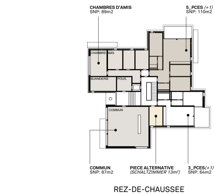
REZ-DE-CHAUSSÉE
