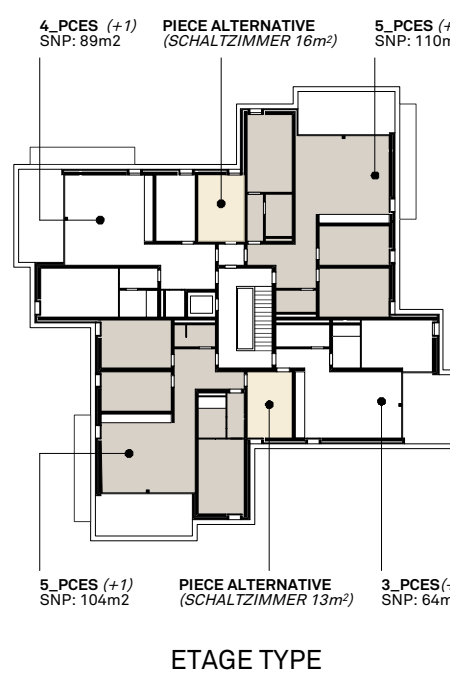
ÉTAGE TYPE
